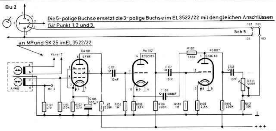
Zusatzverstärker im EL 3522/80 (Stereo-Wiedergabe)
